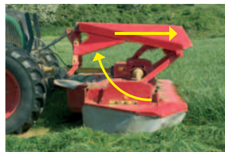
Contour Float - stroj je tažen v nahore umístěném hlavním rámu
