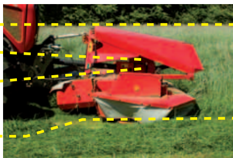
Contour Float - Boční náklon až 12°
