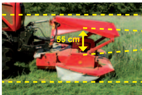
Contour Float - Svislý pohyb až 55 cm
